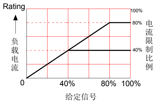
图 7-3a 电流限制
