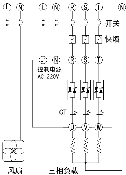
图 3-4a 负载 Y-N 形接线
