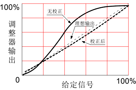
图 7-1 移相
