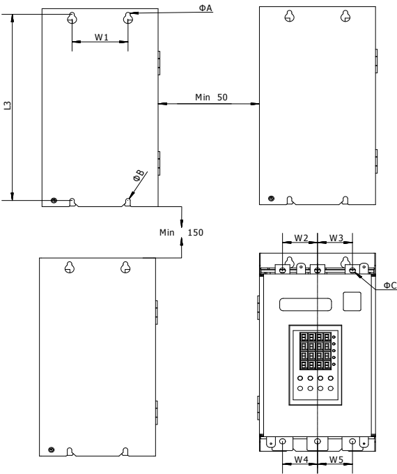
图 3-1 调功器安装示意图
