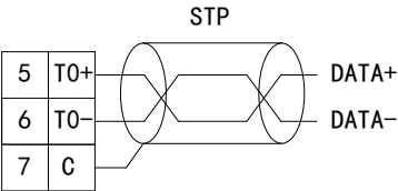
图 3-4 串口接线
