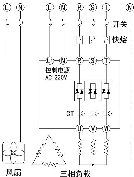
图 3-4b 负载 Y 形或△形接线方式
