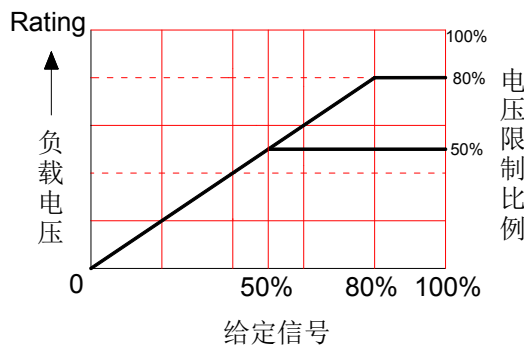
图 7-3b 电压限制
