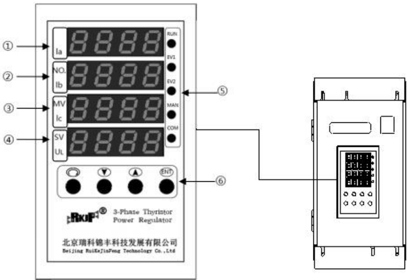
图 4-2 显示面板
