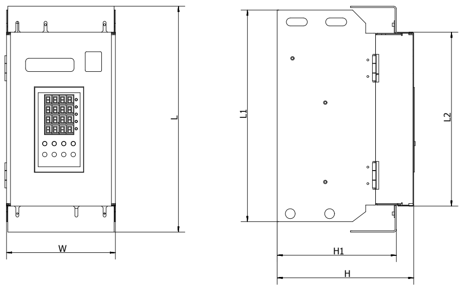
图 3-2 外形尺寸图
