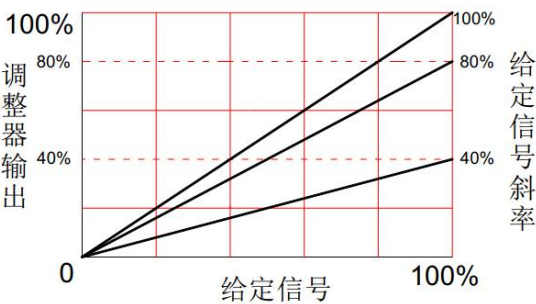
图 7-2a 功率线性限幅
