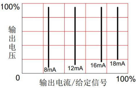
图 7-2b 恒定电流控制
