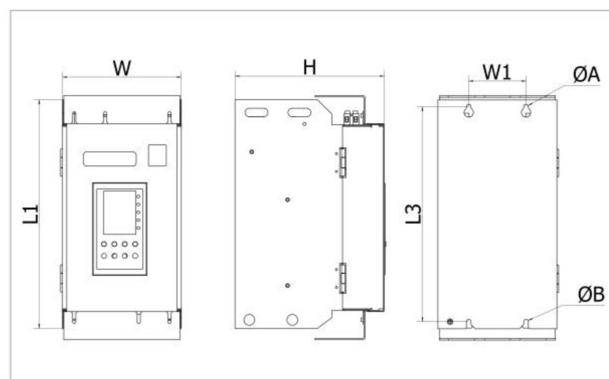
图一 (RKF-5/6-外型及安装图)
