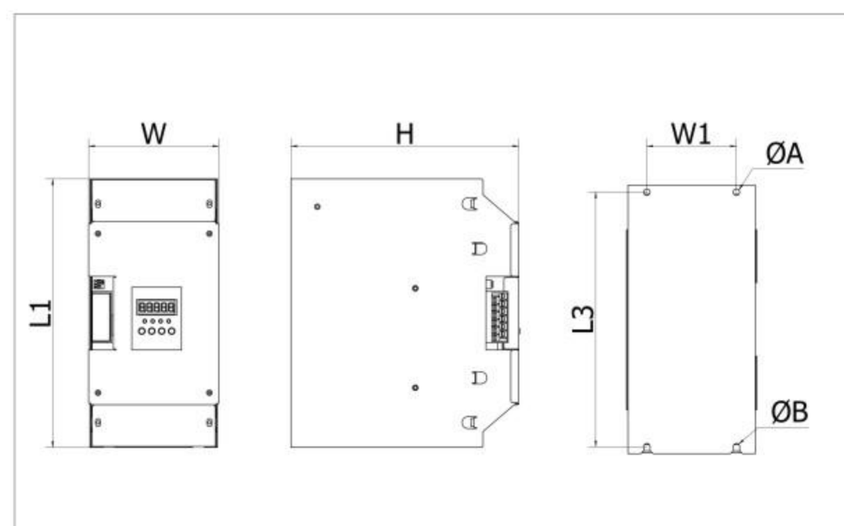
图三 (RKF-A-外型及安装图)
