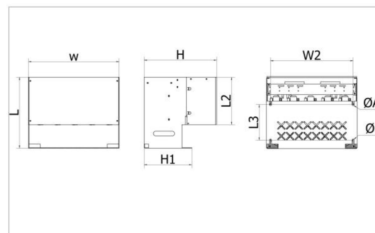
图六 (RKF-M-外型及安装图)
