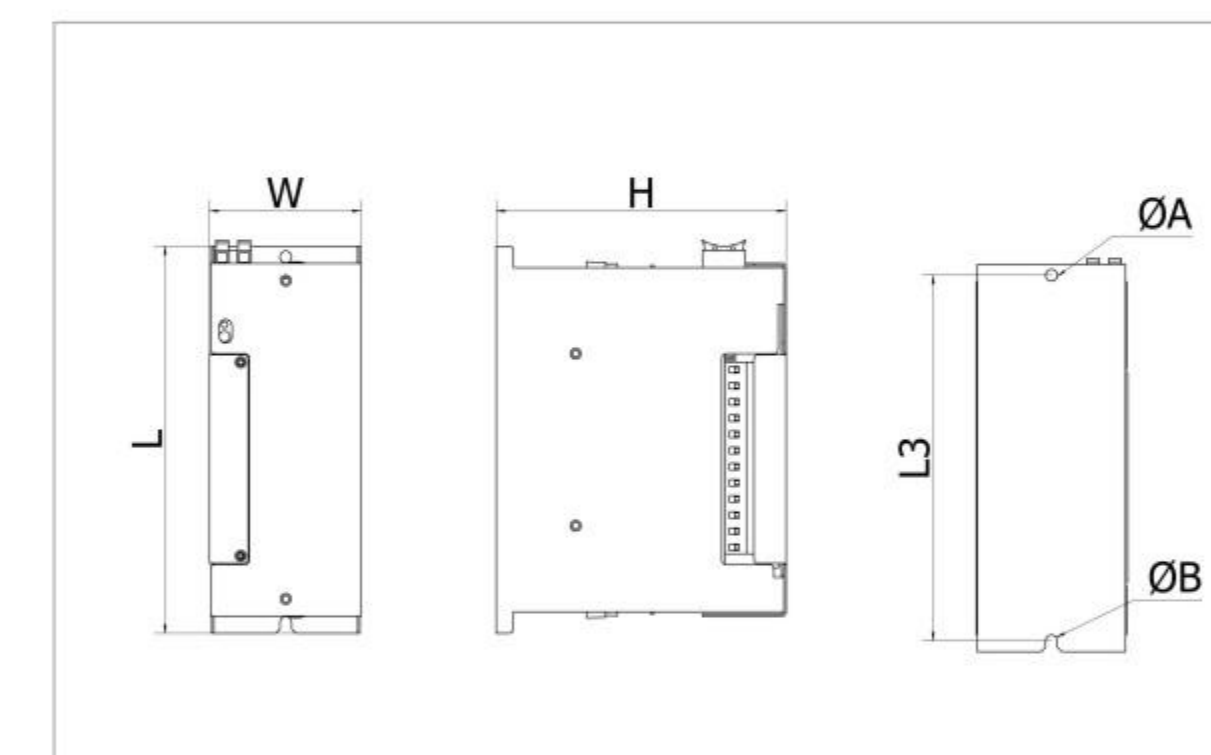
图十二 (RK01AS-外型及安装图)
