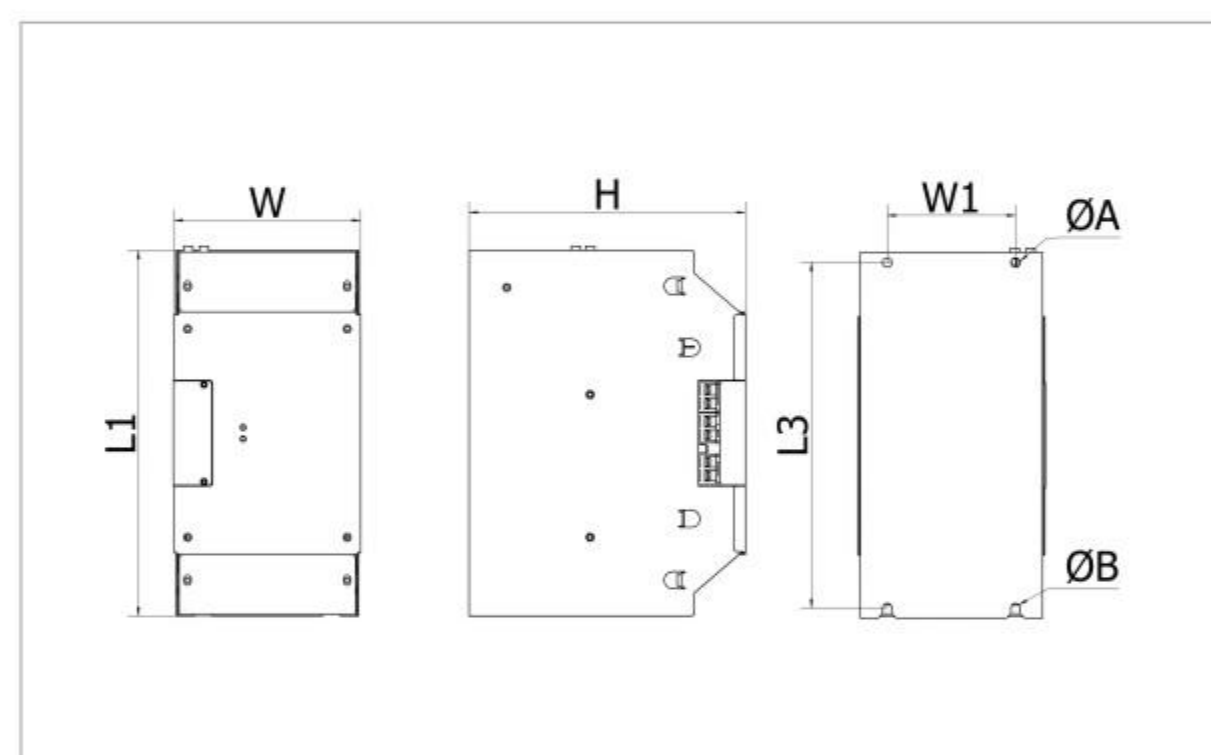
图五 (RKF-G-外型及安装图)
