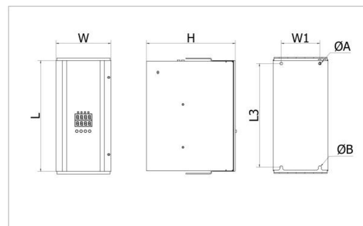
图二 (RKF-4-外型及安装图)
