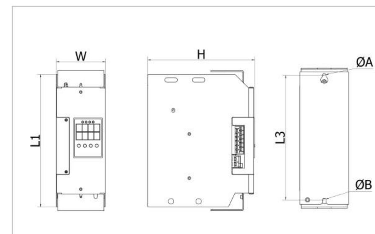
图九 (RKF-2/ZL-外型及安装图)
