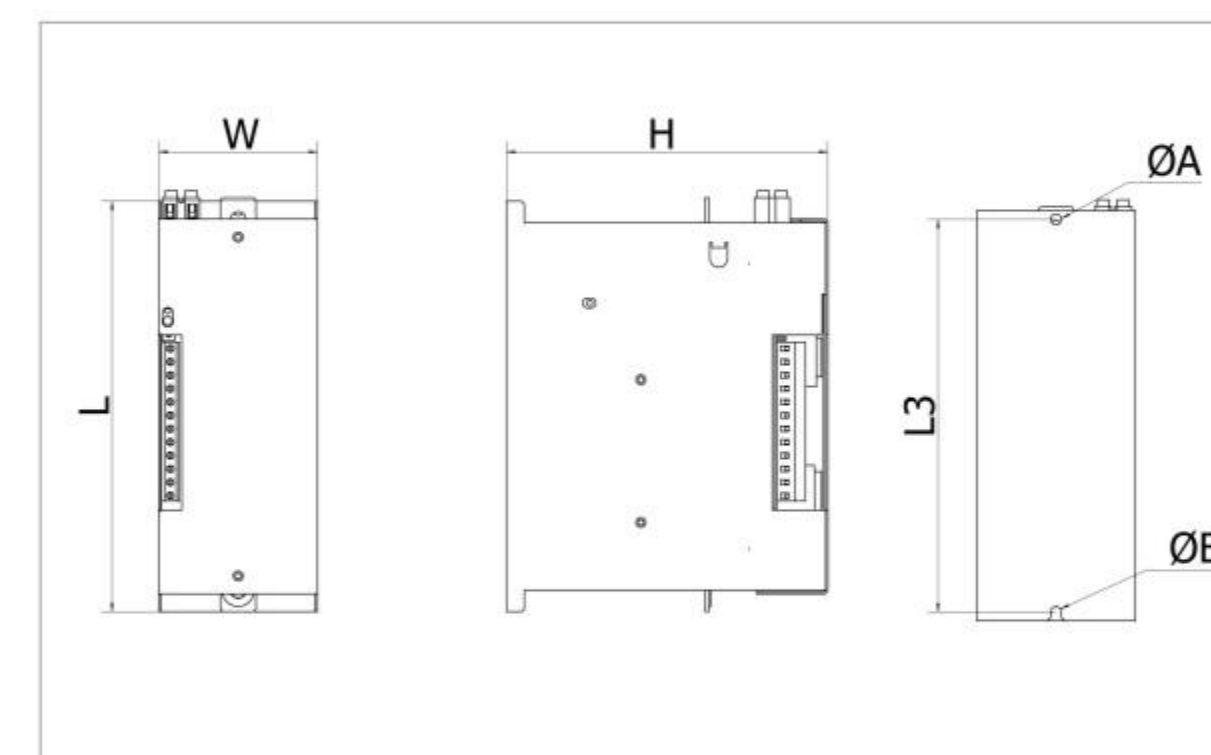
图十一 (RK01A-外型及安装图)
