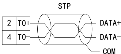
图 3-4 串口接线
